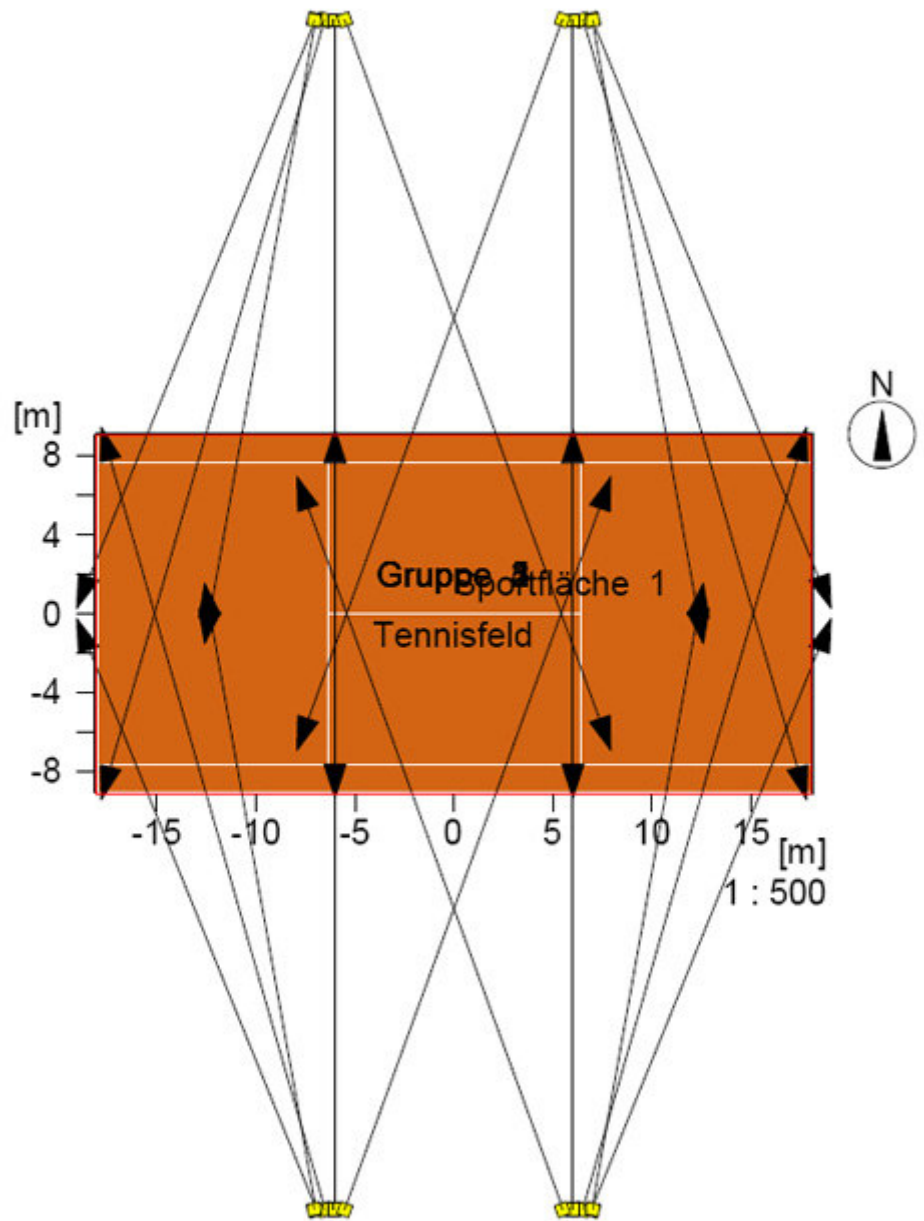
So soll die Beleuchtung der Tennisanlage vonstatten gehen. Bild: Ingenieurbüro Rößler
